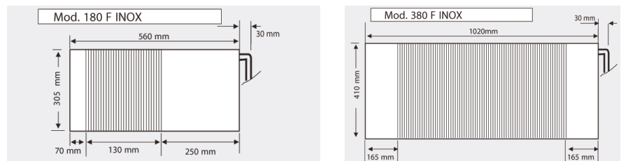
Évaporateur F-inox
