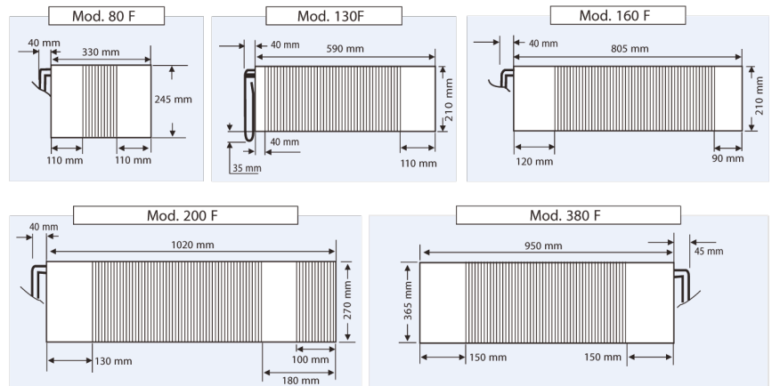
Évaporateur F
